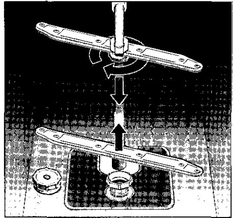
Bras pivotants
